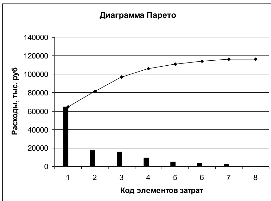
Рисунок 3.3 - Диаграмма Парето
