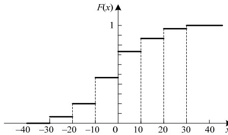
Рис. 19.2. Функция распределения □
